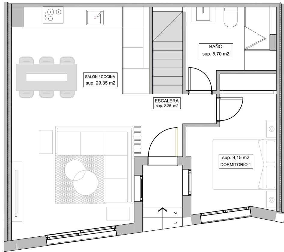
planta baja
