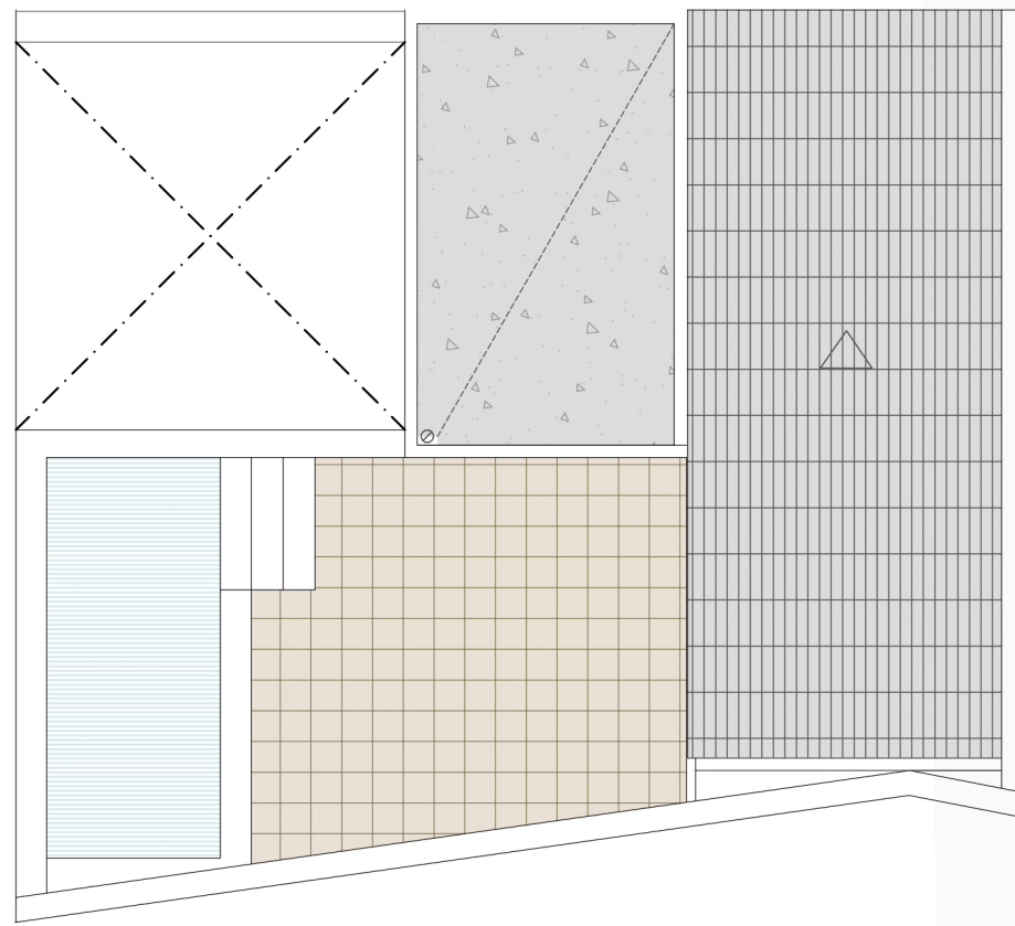
planta cubierta
