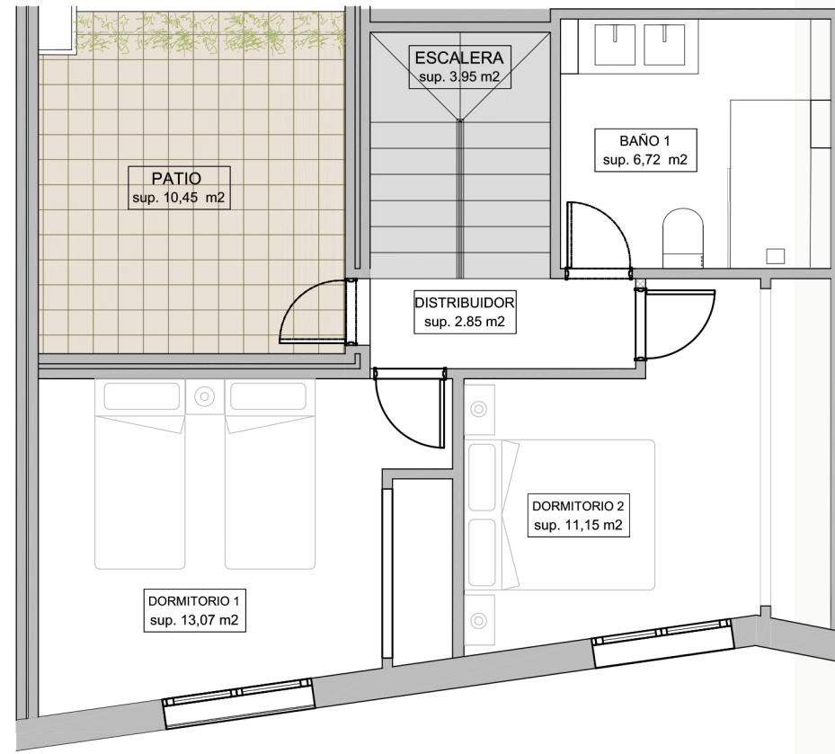
planta primera
