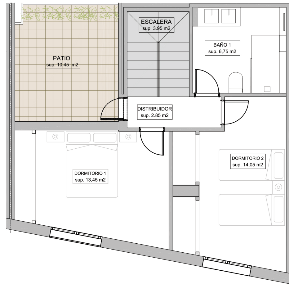
planta primera
