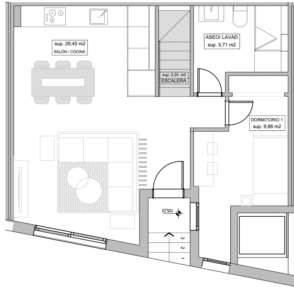
planta baja
