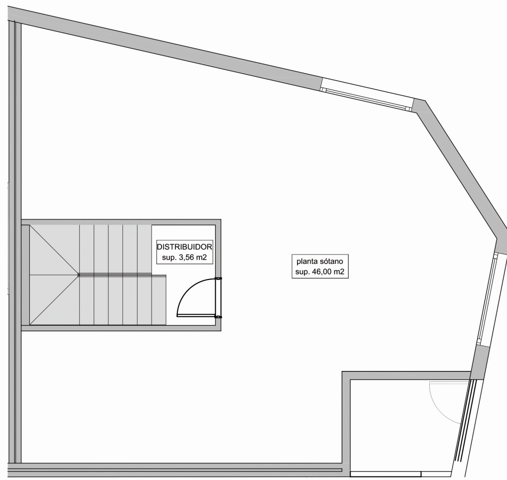
planta sótano
