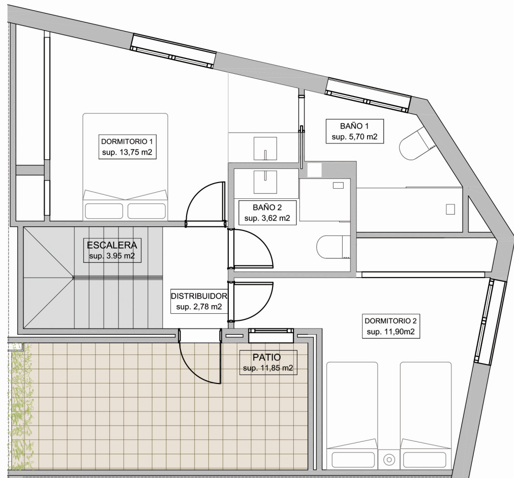
planta primera
