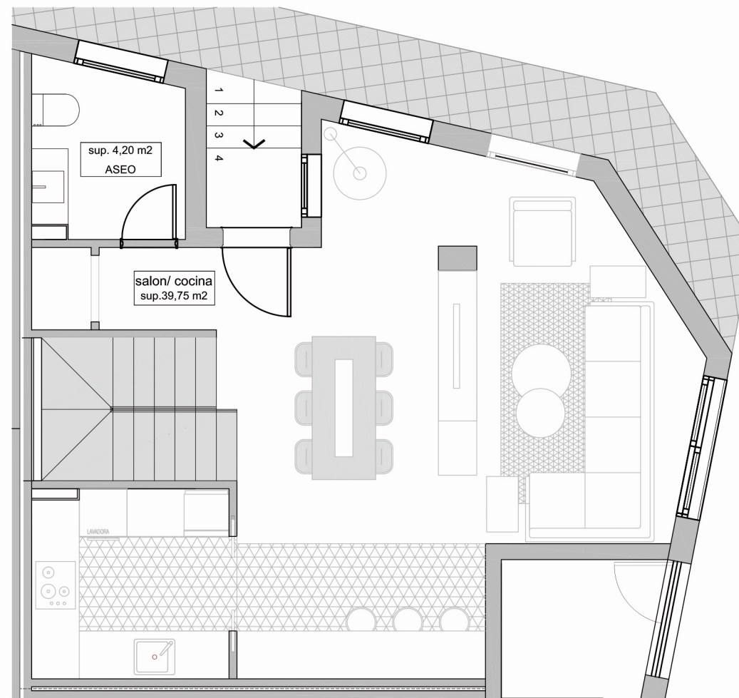
planta baja
