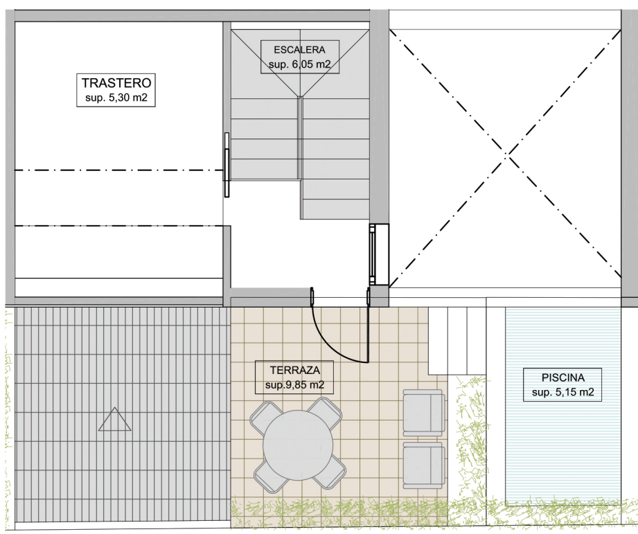
planta castillete - terraza
