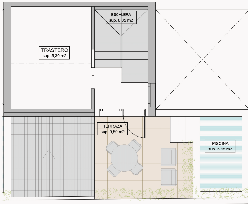
planta castillete - terraza
